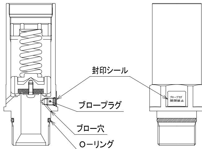
図1 LPR-680Jの構造
